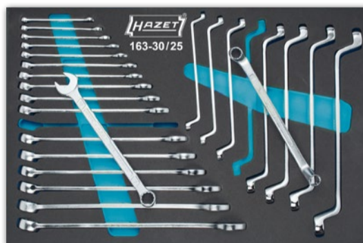
Zestaw kluczy płasko-oczkowych/kluczy oczkowych dwustronnych 163-30/25
